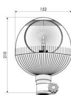
LAMPE H1
